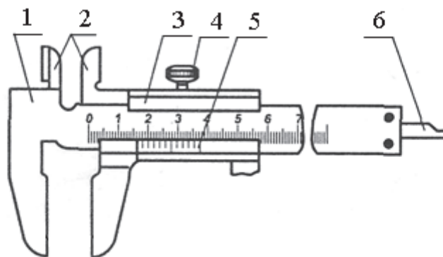
1 – штанга-линейка; 2 – измерительные губки; 3 – рамка; 4 – винт зажима рамки; 5 – нониус; 6 – линейка глубиномера Рисунок 5.1 – Конструкция штангенциркуля типа ШЦ-I
