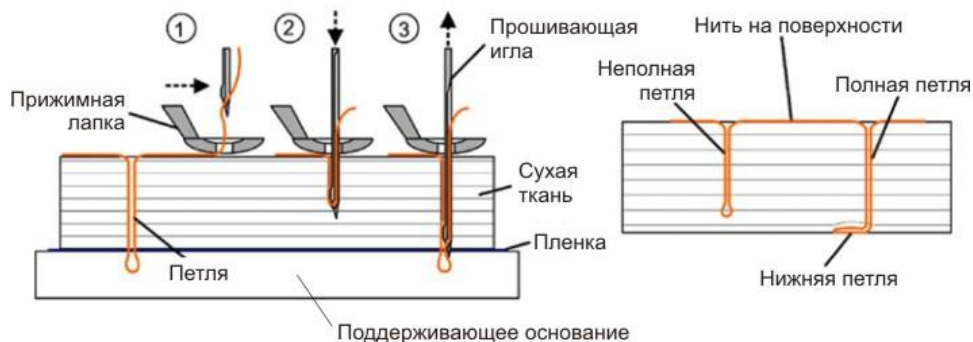
Рисунок 1 – Тафтинговый шов
