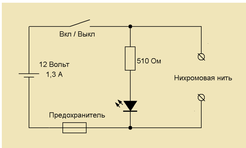
Рисунок 2 – Пример электрической схемы пенорезки
