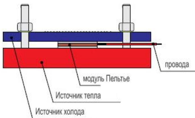
Рисунок 1 Принципиальное строение модульного генератора.
