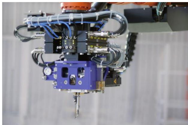
Рисунок 2 - Пример тафтинговой головки для прошивки панелей
