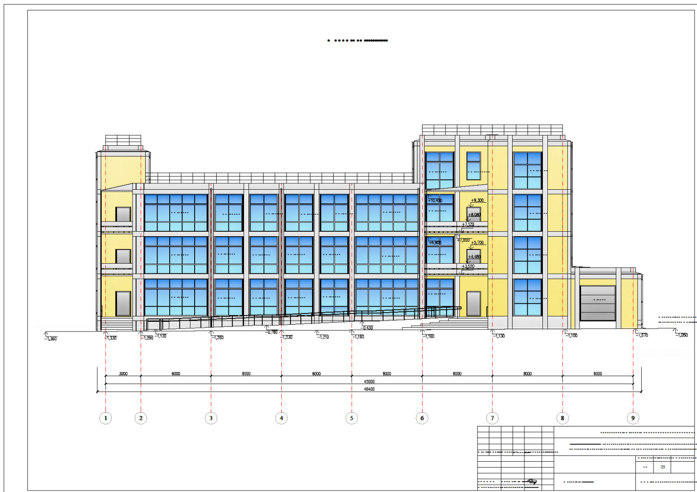
Рисунок 1 – Фасад в осях 1-9
