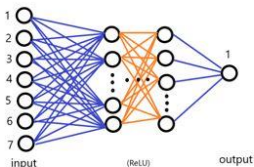
Рисунок 7– Архитектура нейронной сети MLP
