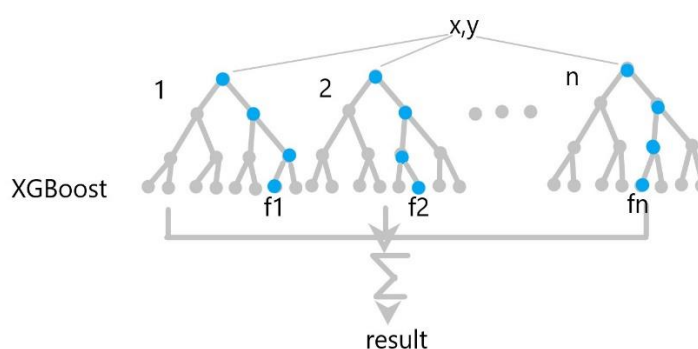
Рисунок 6 - Схема алгоритма XGBoost .
