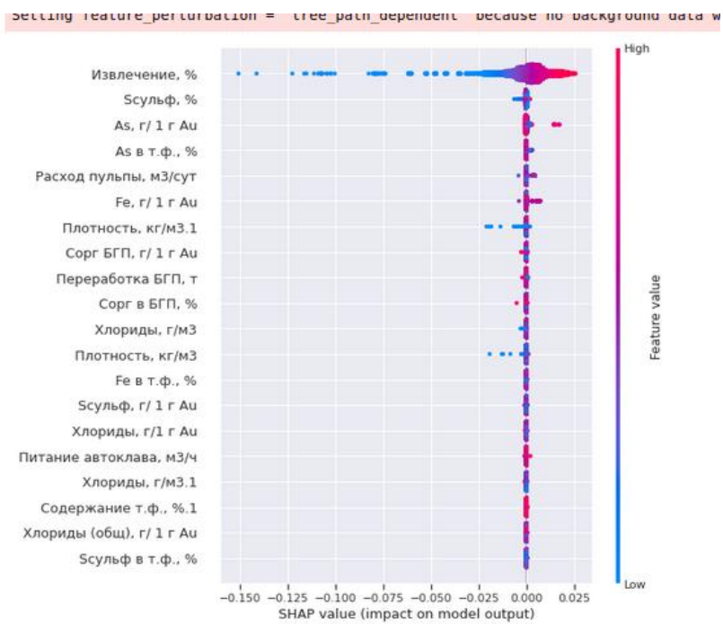
Рисунок 10 – График Шепли
