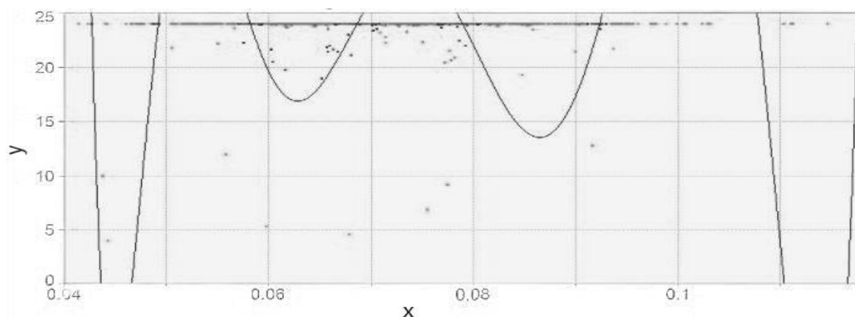
Рисунок 4 – График функции 2
