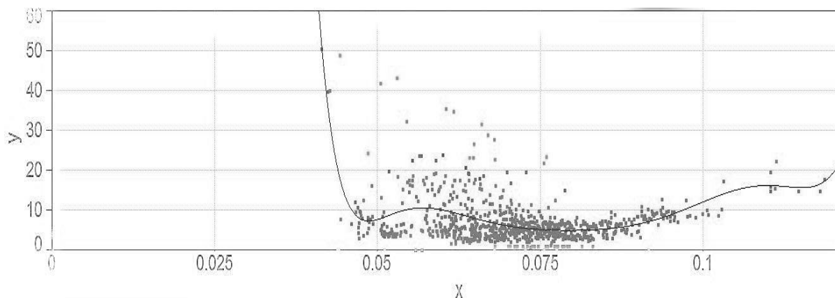
Рисунок 3 – График функции 1
