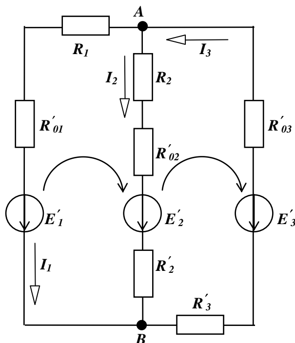
Рис. 2. Схема замещения электрической цепи в примере выполнения задачи 23
