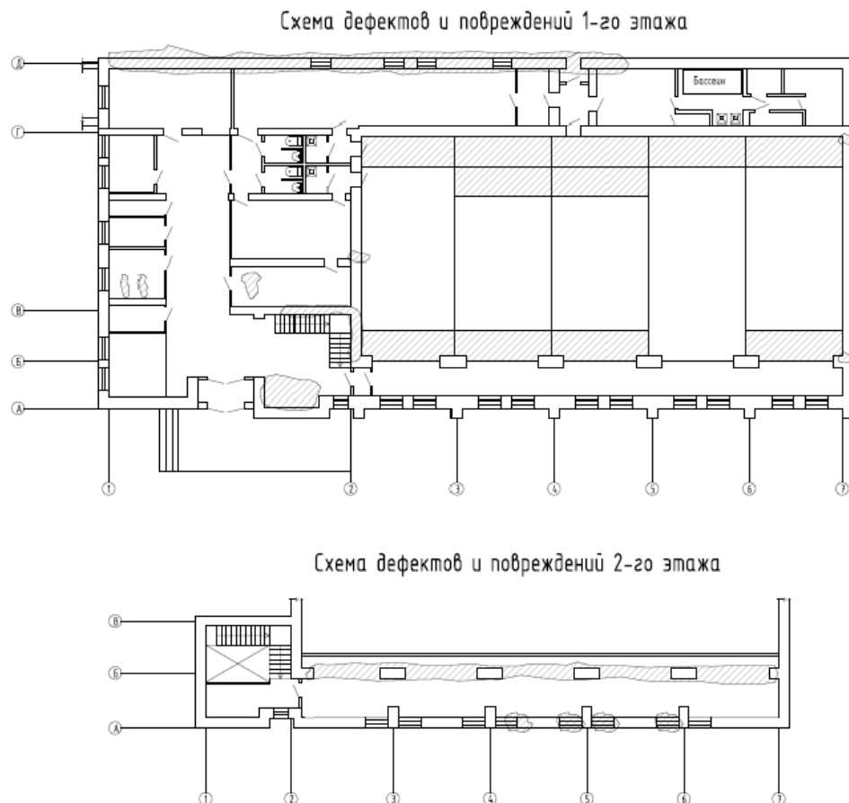
Рис. 1. Картограмма диагностики несущих конструкций сооружения
