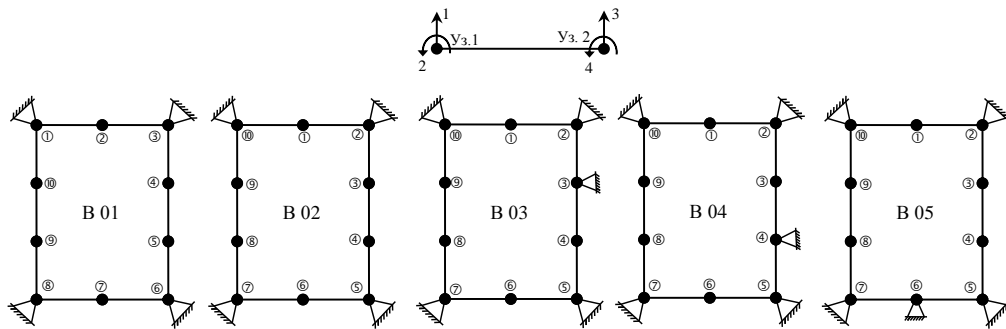
Типовой КЭ с 4 ми узловыми перемещениями (степенями свободы)
