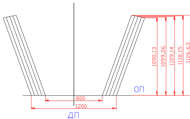
Рисунок 2 – Скег с горизонтальной пяткой переменной ширины
