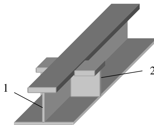
Рисунок 10 – Соединение карлингса с бимсом: 1 - карлингс, 2 - бимс
