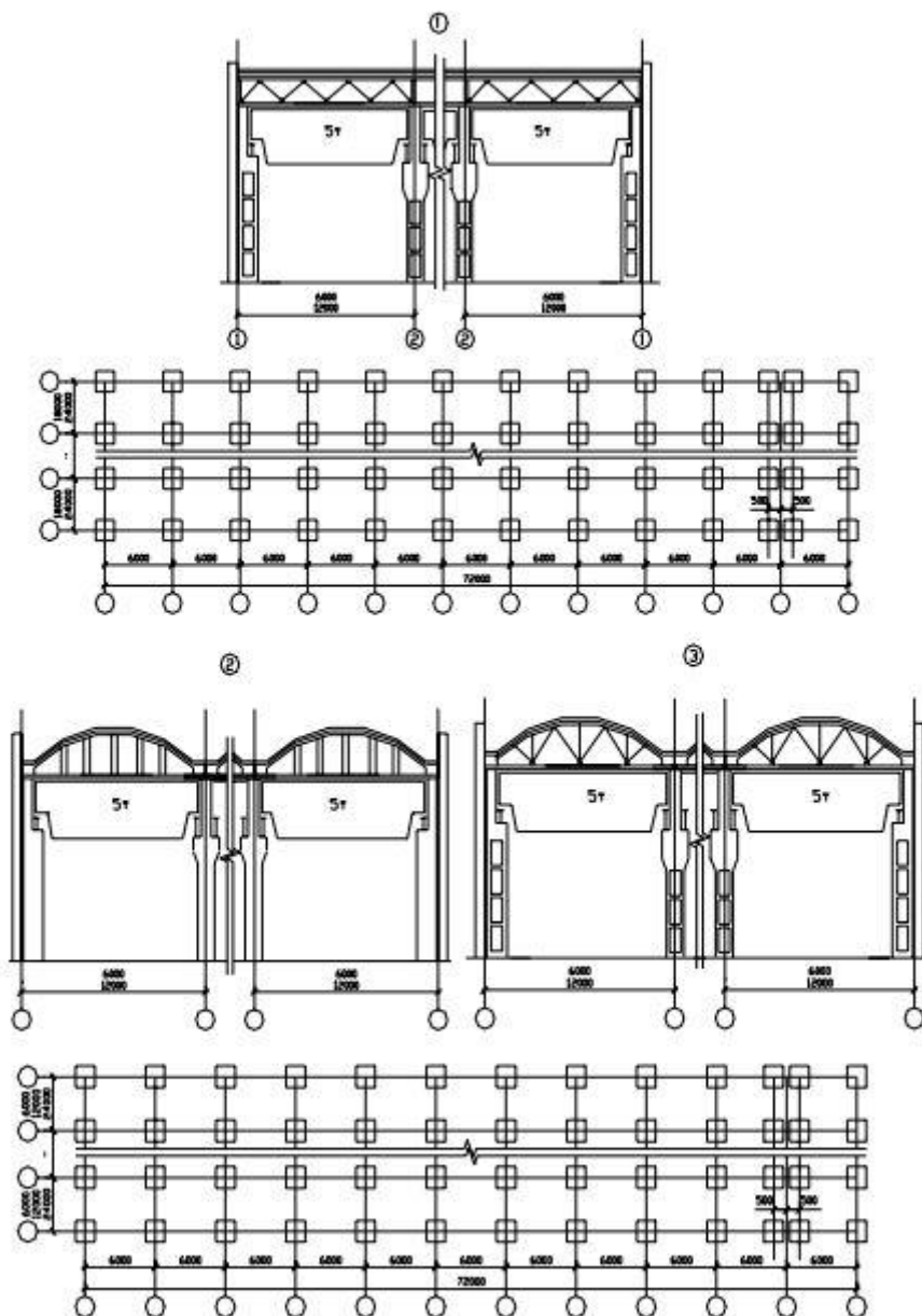
Рисунок 1. Схема зданий
