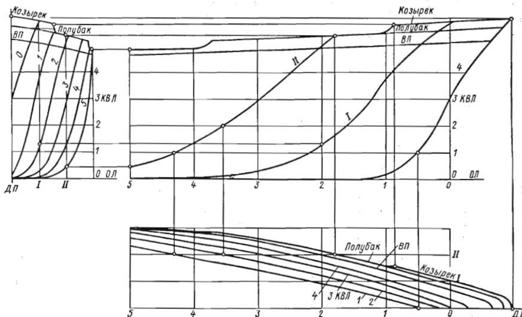
Рисунок 1.5 – Согласование обводов
