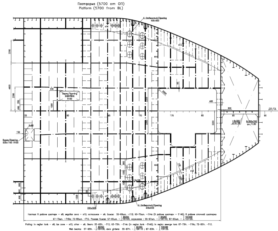
Рисунок 2.1 - Конструктивный чертёж платформы
