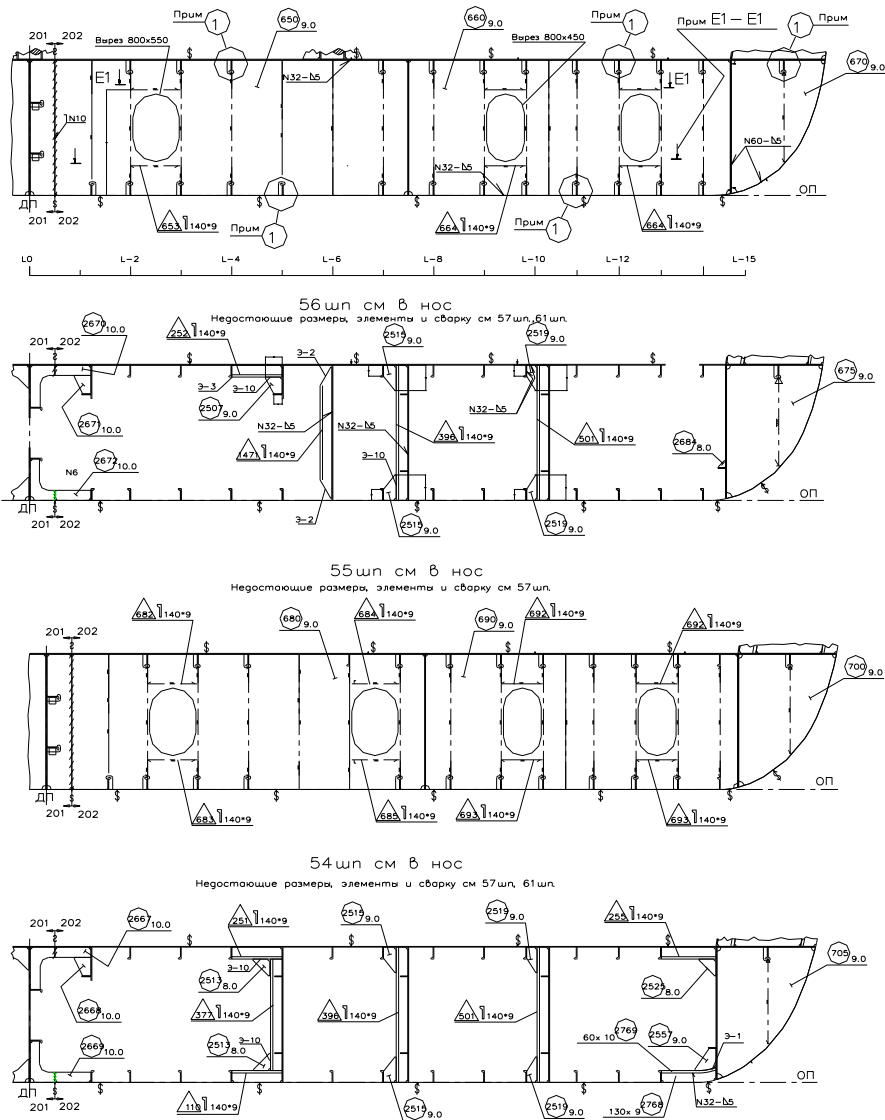
Рисунок 2.1 – Фрагмент конструкции судна
