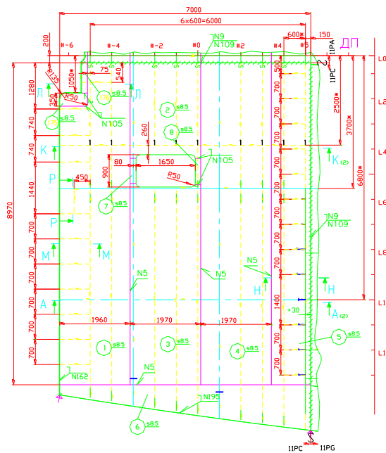
Рисунок 2.3 – План палубы
