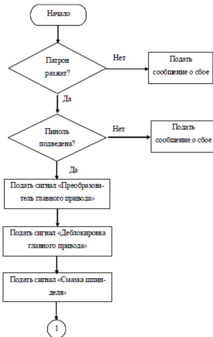
Рис. 1. Алгоритм включения шпинделя
