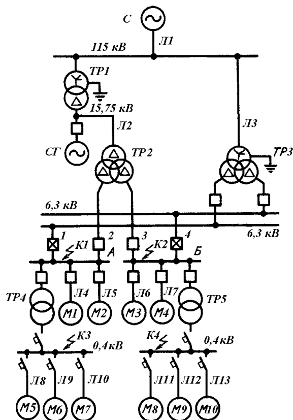
Рис. 1. Часть схемы энерго-
