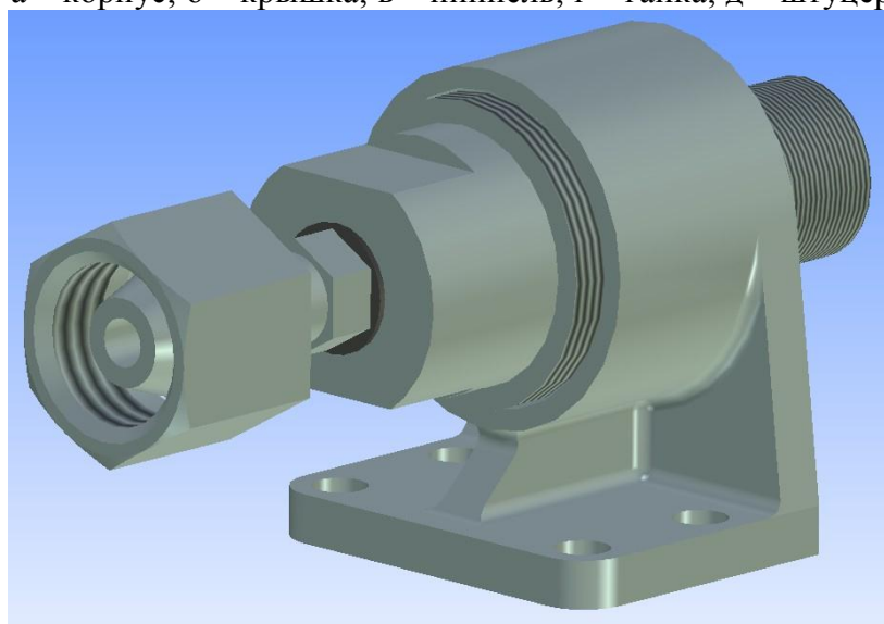
Рисунок 5 – Трехмерные модели деталей сборочного узла: а – корпус; б – крышка; в – ниппель; г – гайка; д – штуцер
