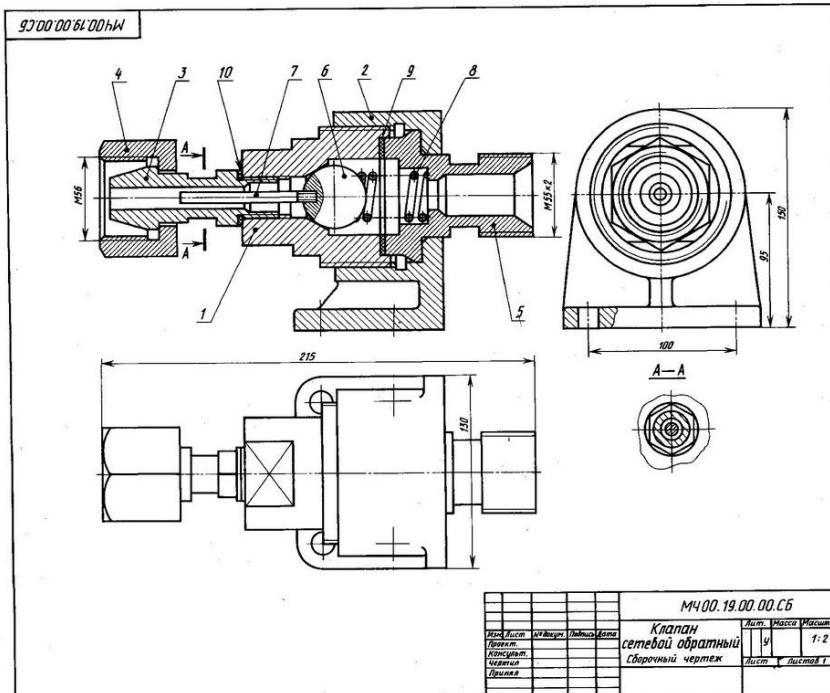
Рисунок 4 – Вариант сборочного чертежа для моделирования.
