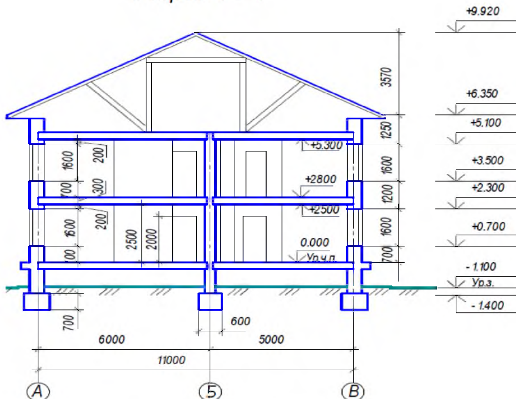
Рисунок 2. Разрез здания
