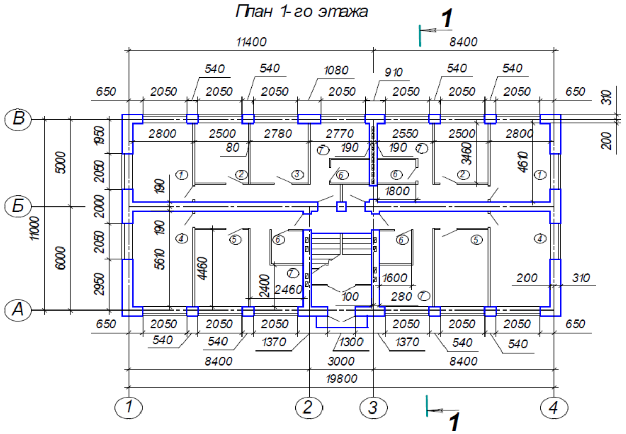
Рисунок 1. План первого этажа здания Разрез 1 - 1
