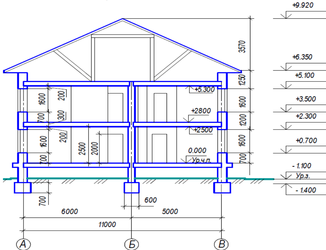
Рисунок 2. Разрез здания
