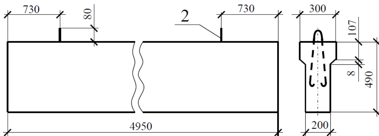
Рисунок 4. Опалубочный чертеж фундаментной балки
