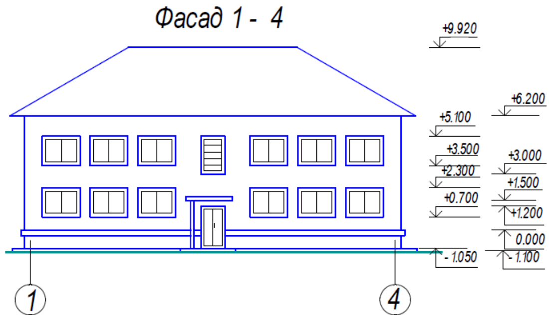
Рисунок 3. Фасад здания
