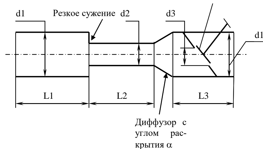
Б. Схема короткого трубопровода
