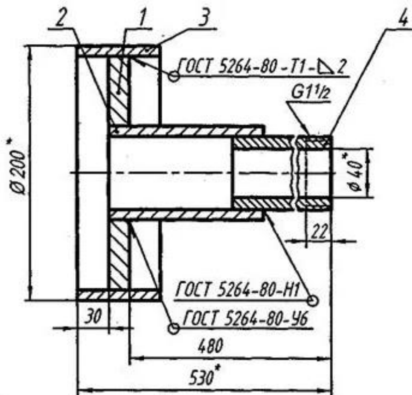
Чертеж 4. Опора.
