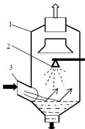
Рис. 3 Полный форсуночный скруббер
