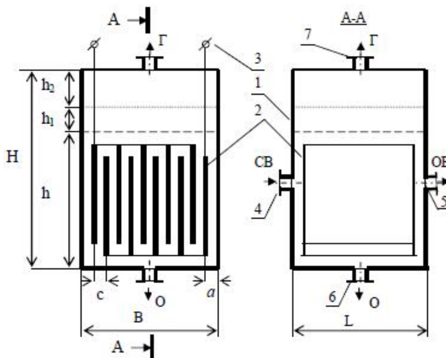
Рис .9. Схема прямоугольного электрокоагулятора.
